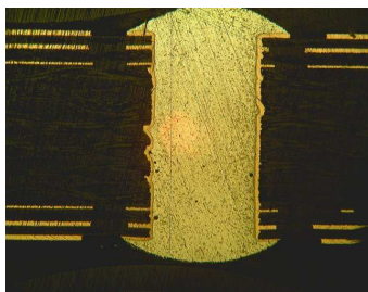
Vertikalt konventionellt snittprov är vanligast förekommande
