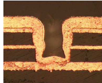
Mikrovia som är ytetsat för mer framträdande korngränser
